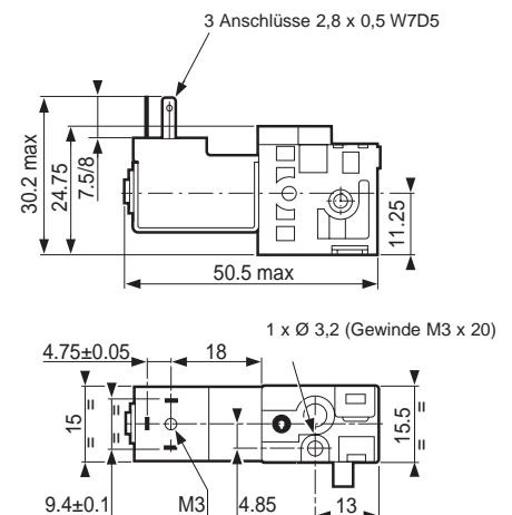
Zwischenbaustein 81 547 5
